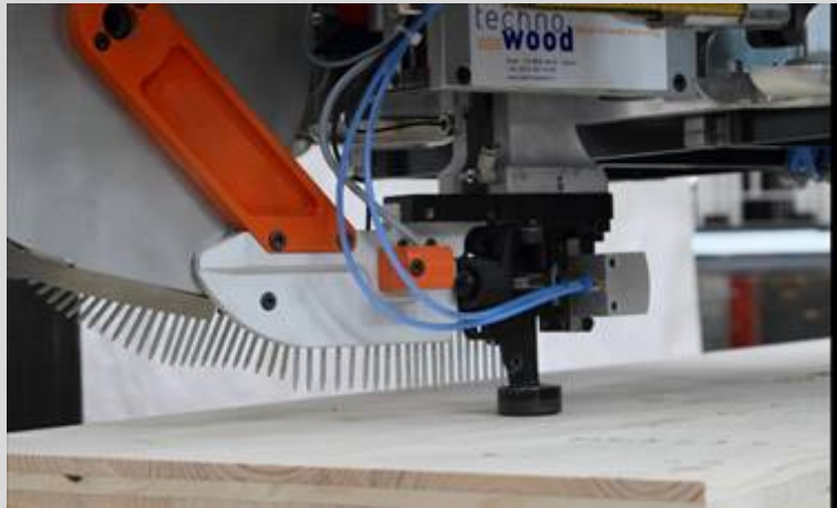
Abb.: E-Modul bietet Platz für bis zu 8 Spezialaggregate (z.B. Nagel-, Klammer- und Fräsaggregate)
